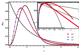
Anderson 模型: 準位間隔分布 Nishigaki et al. 2013
