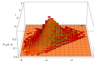
\mathfrak{S}_N の最長・第2増加部分列
