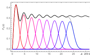
最小固有値分布
