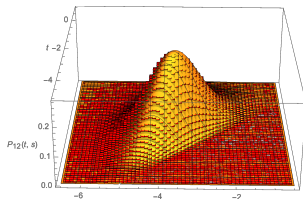
最大・第2固有値
