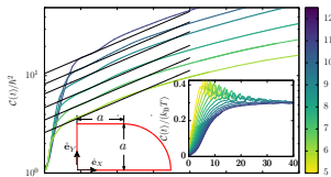
Sinai ビリヤード: 非時間順序積 García-Mata et al. 2022
