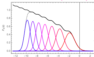
最大固有値分布 (TW 分布)
