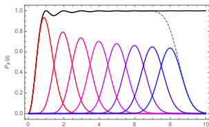
固有値間隔分布
