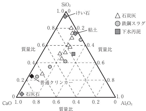
図-1 普通ポルトランドセメントおよび廃棄物の化学組成
