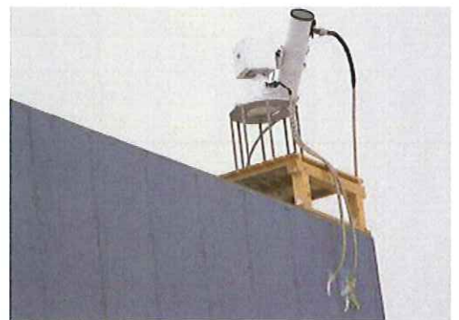
写真8 南極観測で使用した太陽光追尾装置
