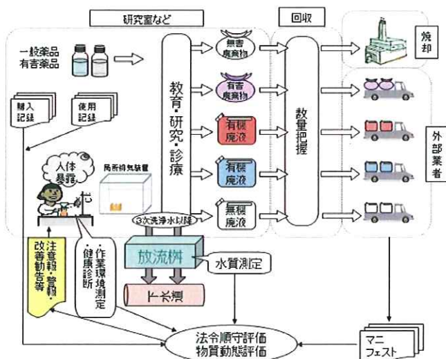
図26 廃棄物フローチャート
