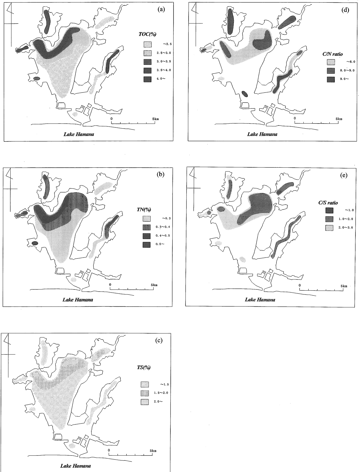
図4. 浜名湖における全有機炭素 (TOC : a) 濃度, 全窒素 (TN : b) 濃度, 全イオウ (TS : c) 濃度, TOC/TN (C/N : d) 比, TOC/TS (C/S : e) 比の堆積物表層分布
