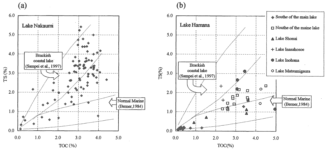
図6. 中海 (a) および浜名湖 (b) における TOC-TS クロスプロット Fig.6 TOC-TS crossplots for Lake Nakaumi (a) and Lake Hamana (b)
