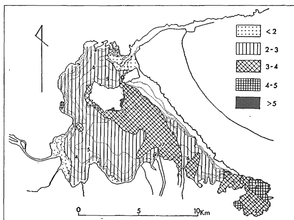
図 8 . 干拓工事による堤防の建設以前の中海の TOC 濃度分布 (小野・小野寺, 1976)
