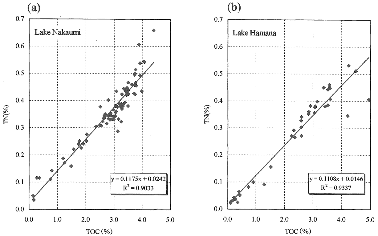
図 5. 中海 (a) および浜名湖 (b) における TOC-TN クロスプロット Fig.5 TOC-TN crossplots for Lake Nakaumi (a) and Lake Hamana (b)
