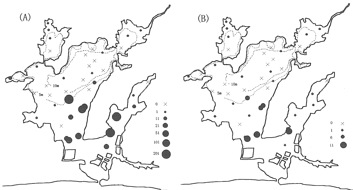
図 2. 貝形虫の産出頻度 (殻数/100cc) (A) と種数分布 (種数/サンプル) (B)
