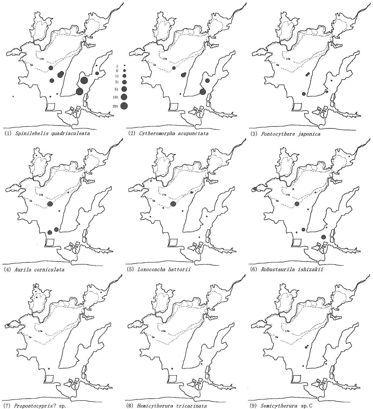
図 6. 浜名湖における貝形虫種分布 Fig.6. Distribution of ostracod species in Lake Hamana.
