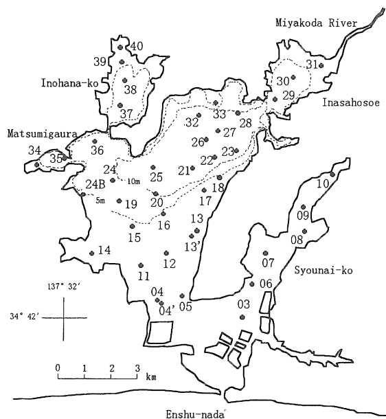
図 1. 浜名湖調査地点
