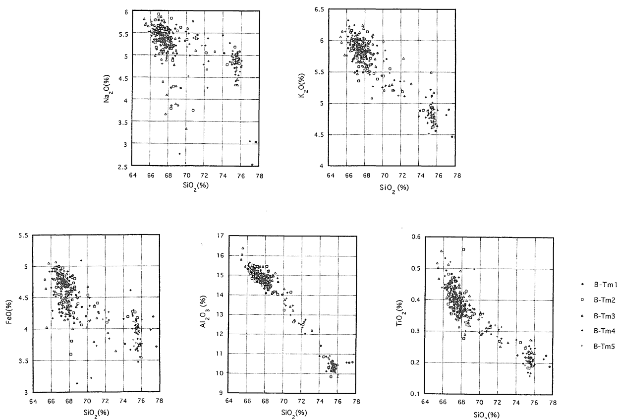
図5 白頭山－苦小牧火山灰 (B-Tm) の火山ガラス分析試料 (B-Tm1, b-Tm2, b-Tm3, B-Tm4, B-Tm5) の \text{SiO}_2 - \text{Na}_2\text{O} , \text{SiO}_2 - \text{K}_2\text{O} , \text{SiO}_2 - \text{FeO} , \text{SiO}_2 - \text{Al}_2\text{O}_3 , \text{SiO}_2 - \text{TiO}_2 の関係図
